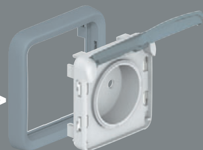
3/ Opětovně nasad'te rámeček na krabici nebo montážní desku
