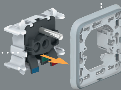
2/ Uchycení mechanismu ze spodní strany
