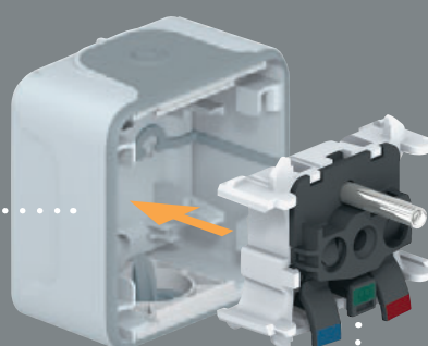
2/ Uchycení mechanismu z čelní strany
