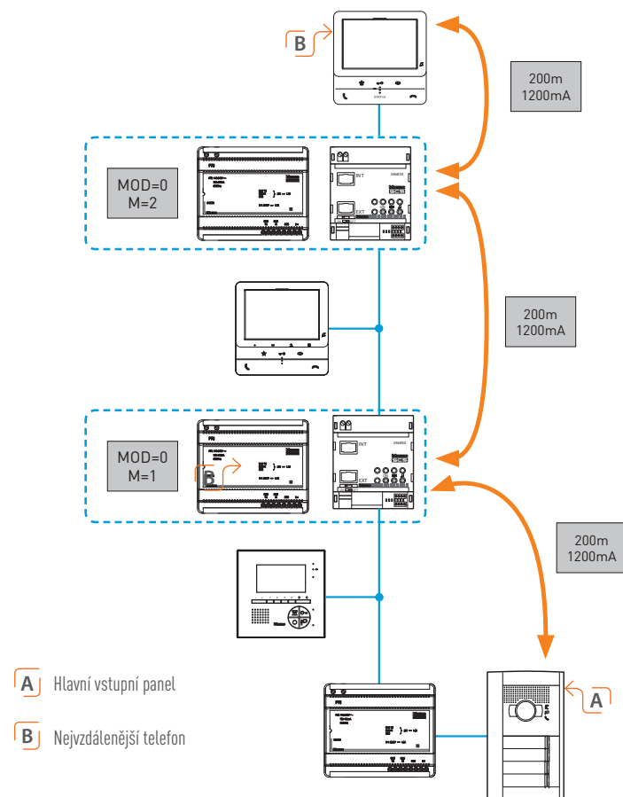
Blokové schéma
